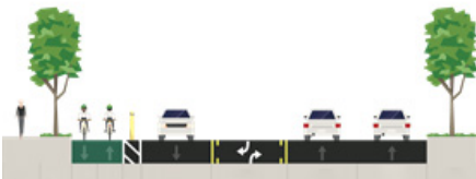
Cắt ngang của làn đường dành cho xe đạp được đề xuất
